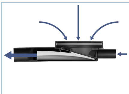
2 När vatten strömmar in i brunnen öppnas membranet och vattnet rinner igenom.
